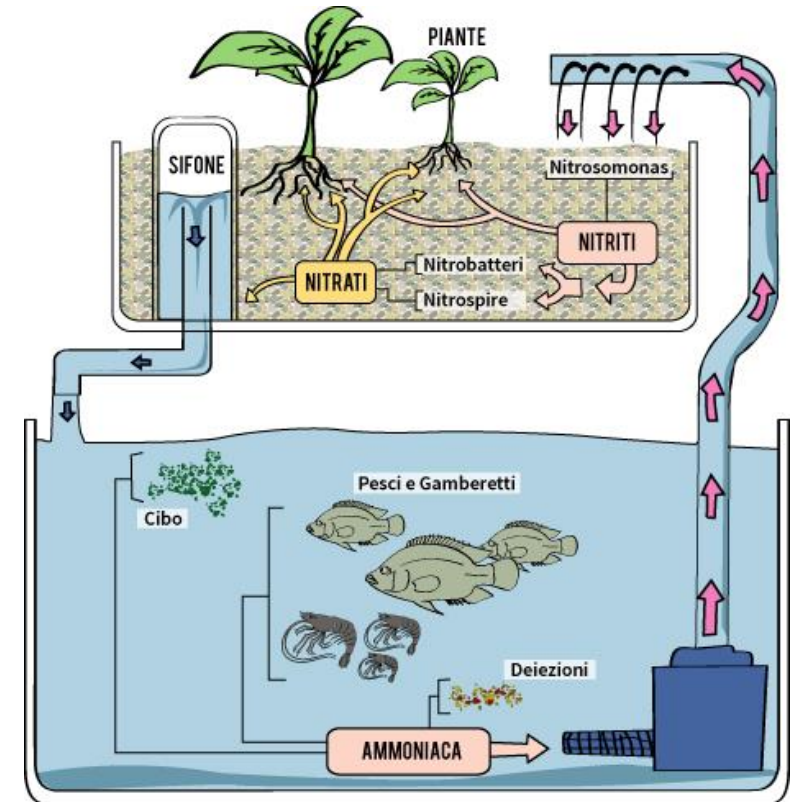
Schema Acquaponica
